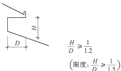
图1 眺台下开口净高度 H 与深度 D 的比值
