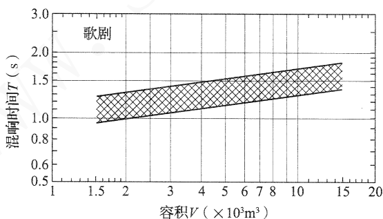
图 3.3.1-1 歌剧、舞剧剧场对不同容积 V 的观众厅,在频率 500~1000Hz 时满场的合适混响时间 T 的范围
